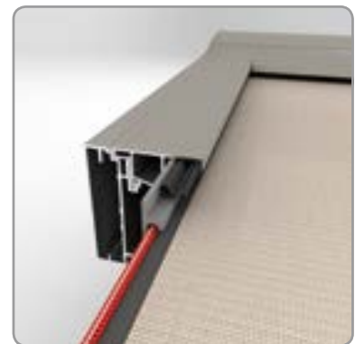
Führung: Fixscreen® Technologie
