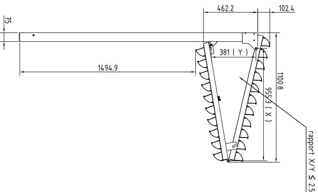
VUE LATÉRALE
