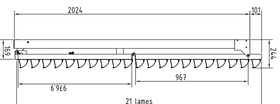
VUE LATÉRALE
