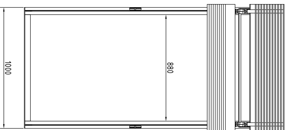
VOORAANZICHT
