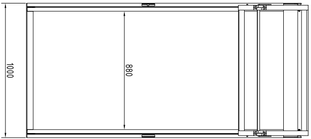
VOORANZICHT
